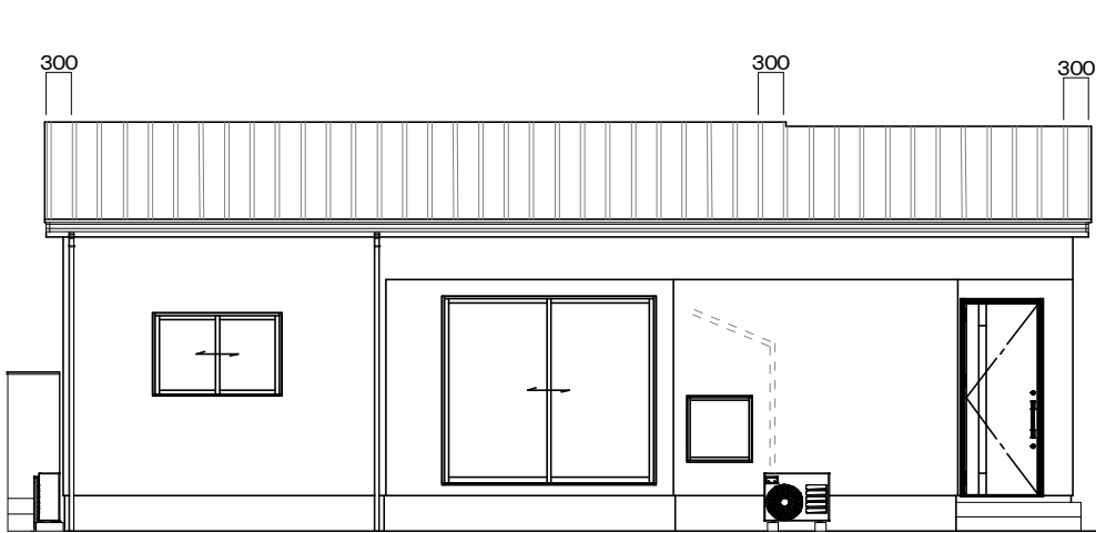
南側立面図
