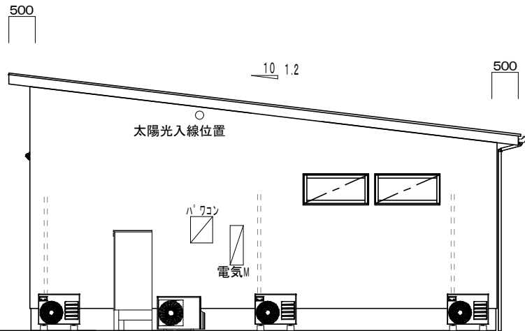
西側立面図
