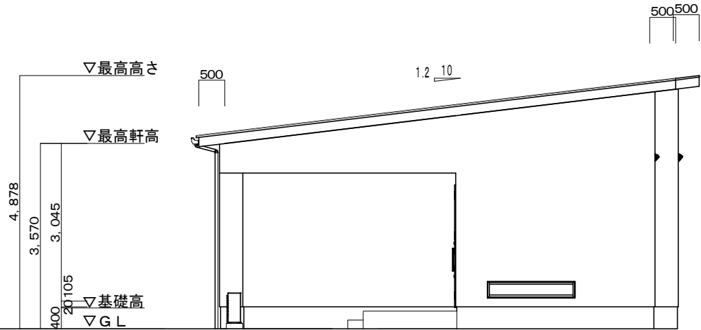
東側立面図
